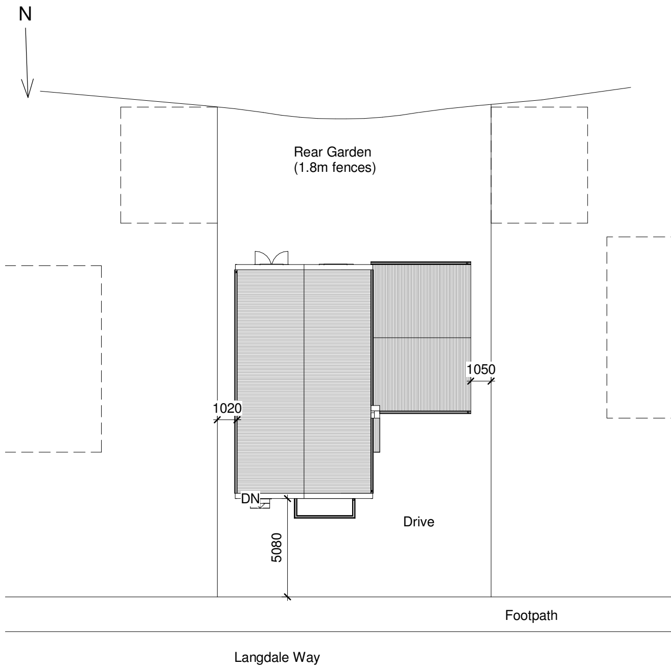
1 Site 1 : 200
